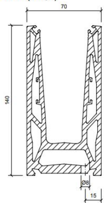
B-B (1:1,5)
