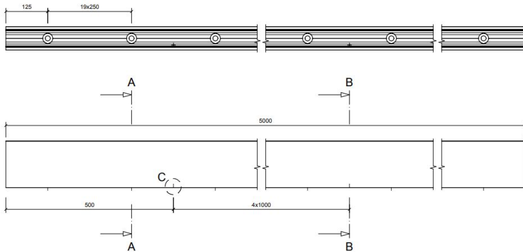
Detail C (1:1,5)
